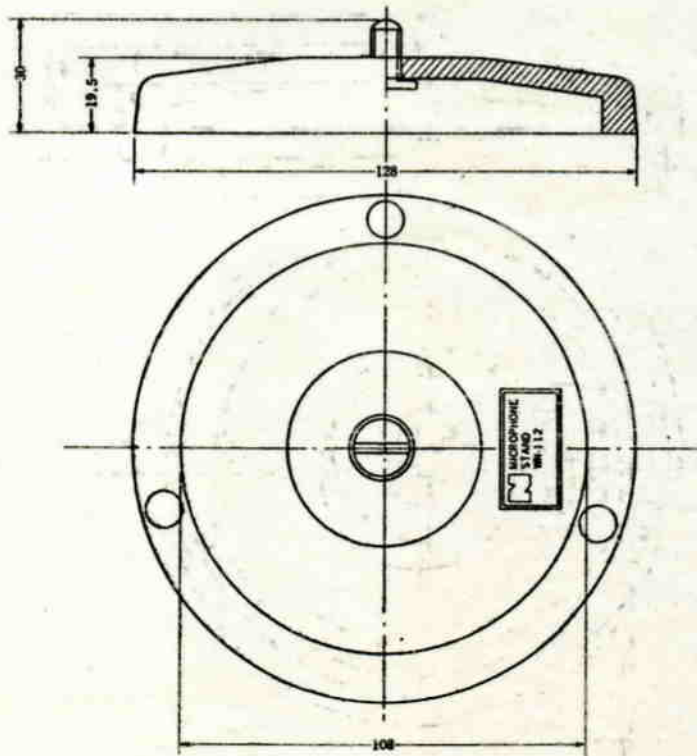
■WN-112寸法図
