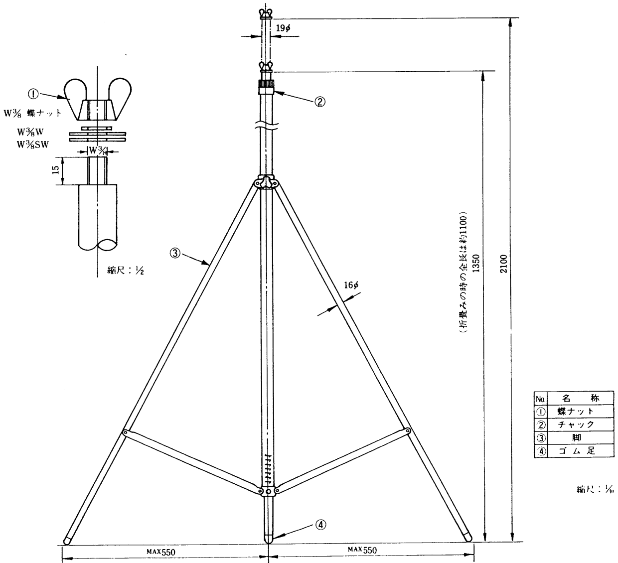
■ WN-900A 外観寸法図
