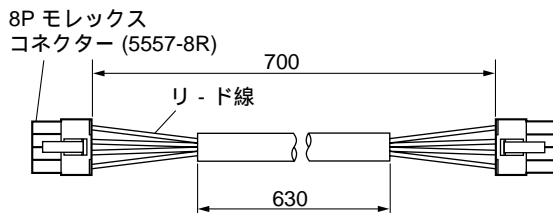
8芯モレックスケーブル
