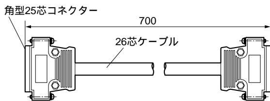
角型25芯D-Subケーブル
