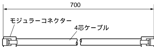
4芯モジュラーケーブル
