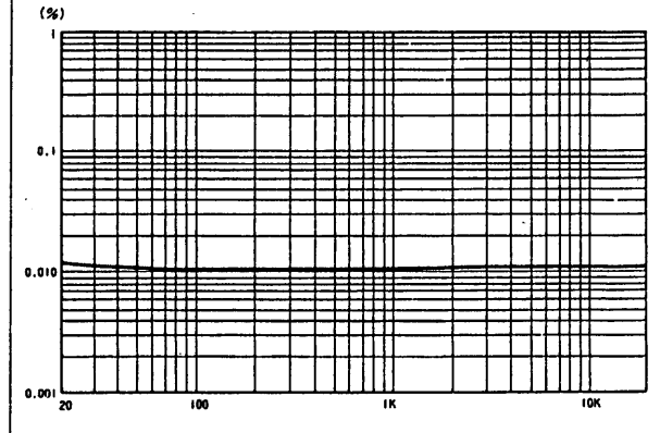
全高調波歪率 モノインプット～マトリクスアウト
