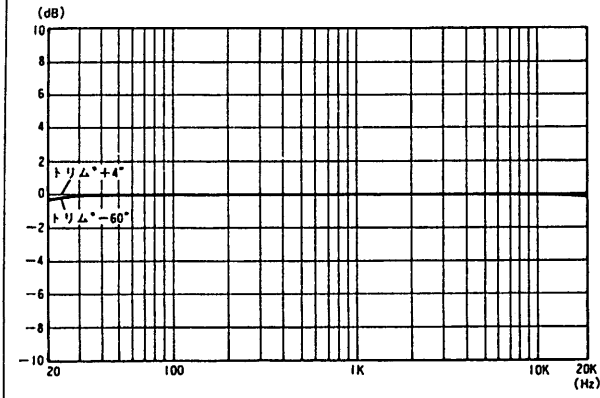
周波数特性 モノインプット～マトリクスアウト
