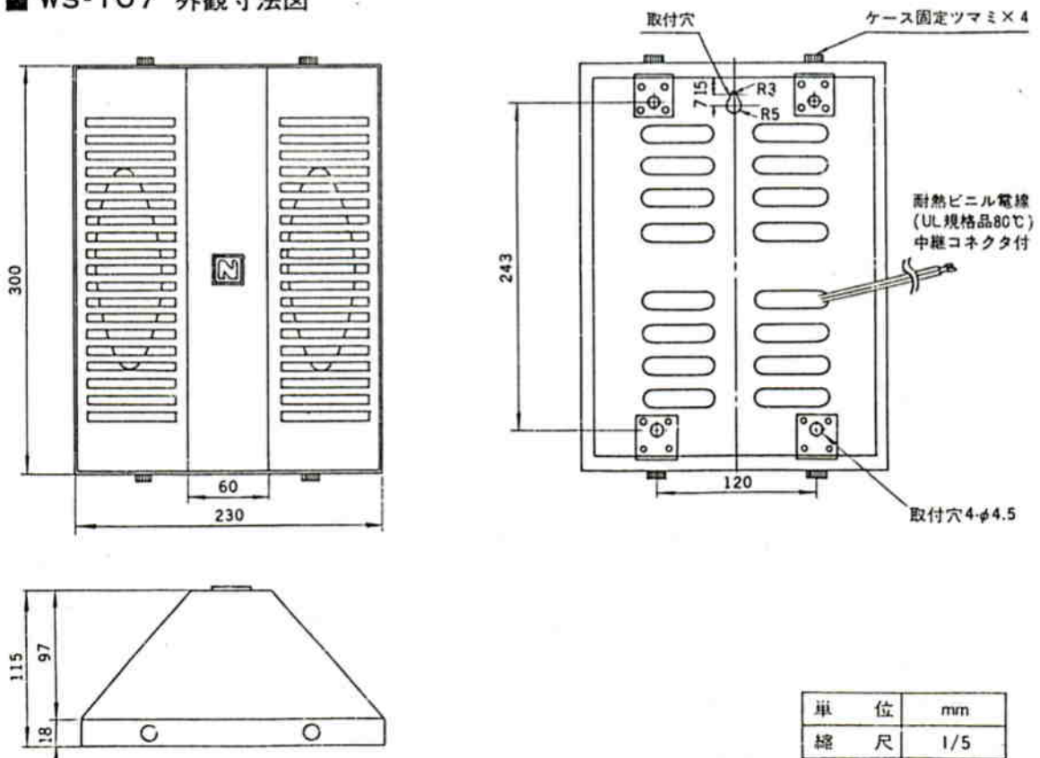
■ WS-107 外観寸法図
