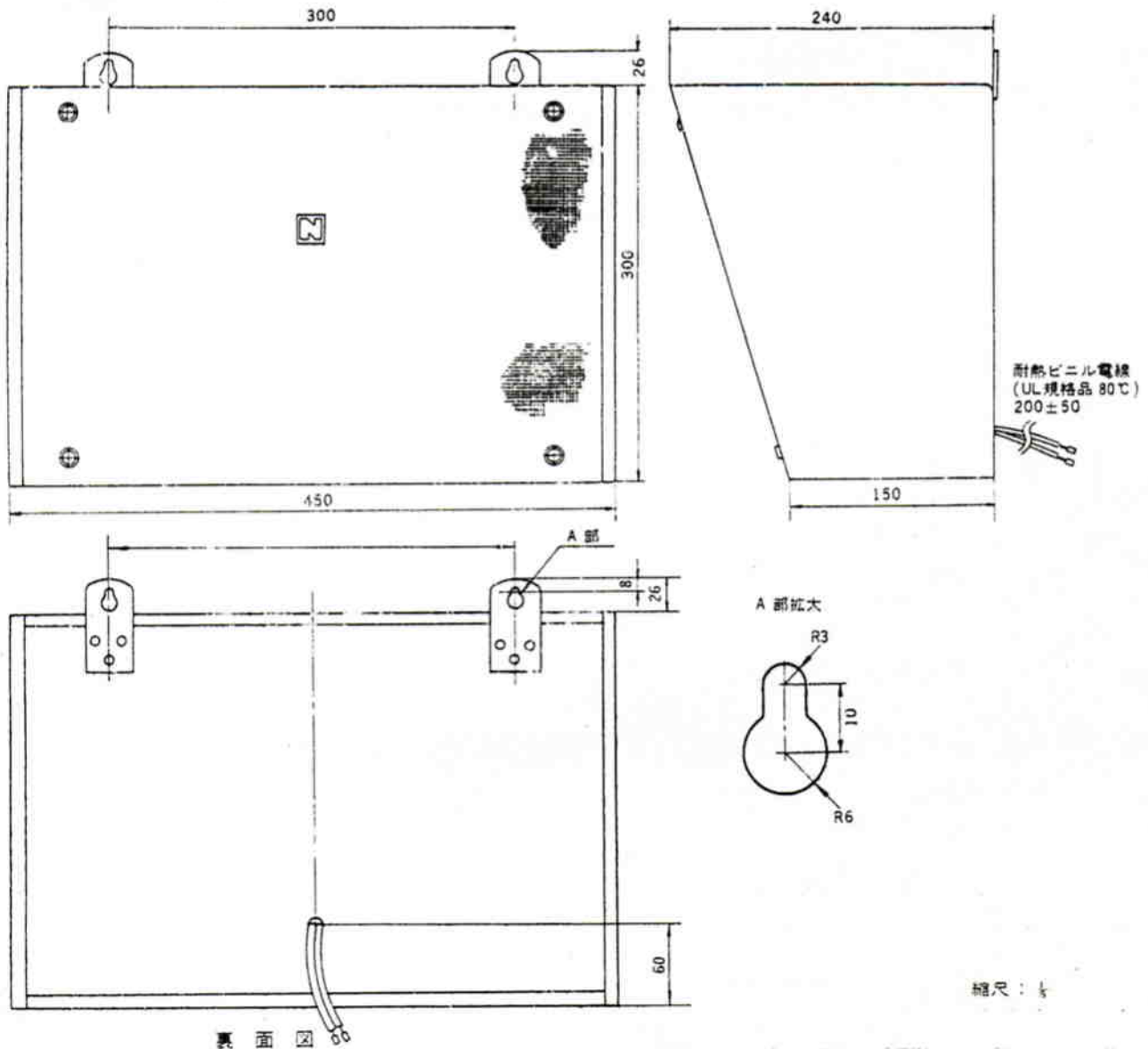
WS-113 外観寸法図
