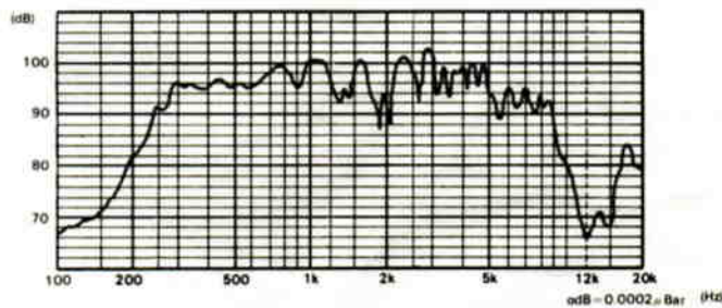
標準周波数特性表
