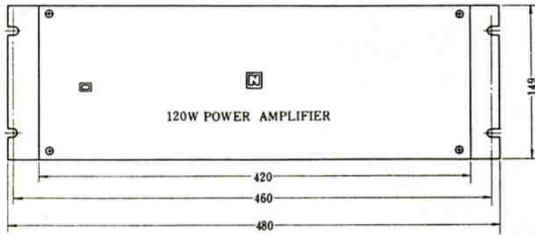
正面図
