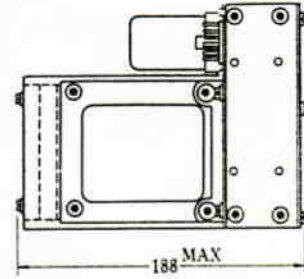
側面図 (ロックマウント型)
