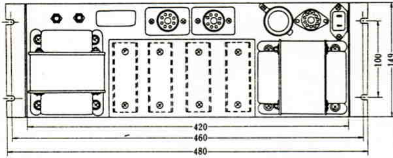
背面図
