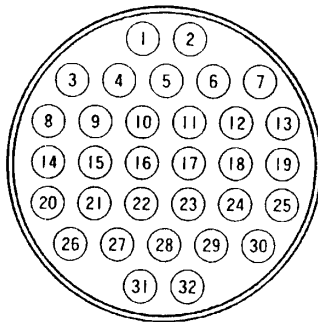
32ピンコネクタ
