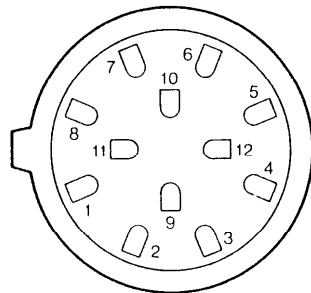
12ピンコネクタ
