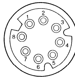
8ピンコネクタ
