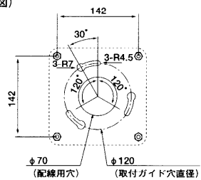
取付金具寸法図 (参考図)
