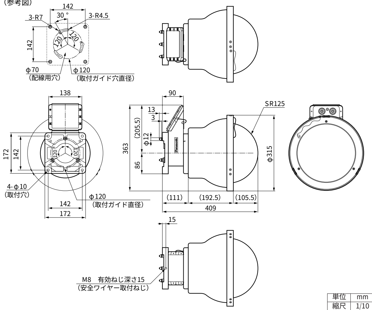
取付金具穴寸法図 (参考図)
