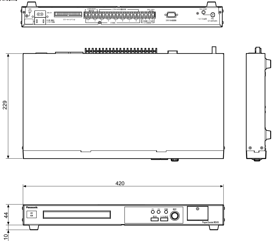
ラックマウント金具 WQ-LA44S 外觀寸法図 (別売品、1セット2個)
