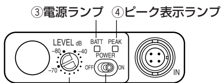
②入力感度調節ボリューム ①電源スイッチ
