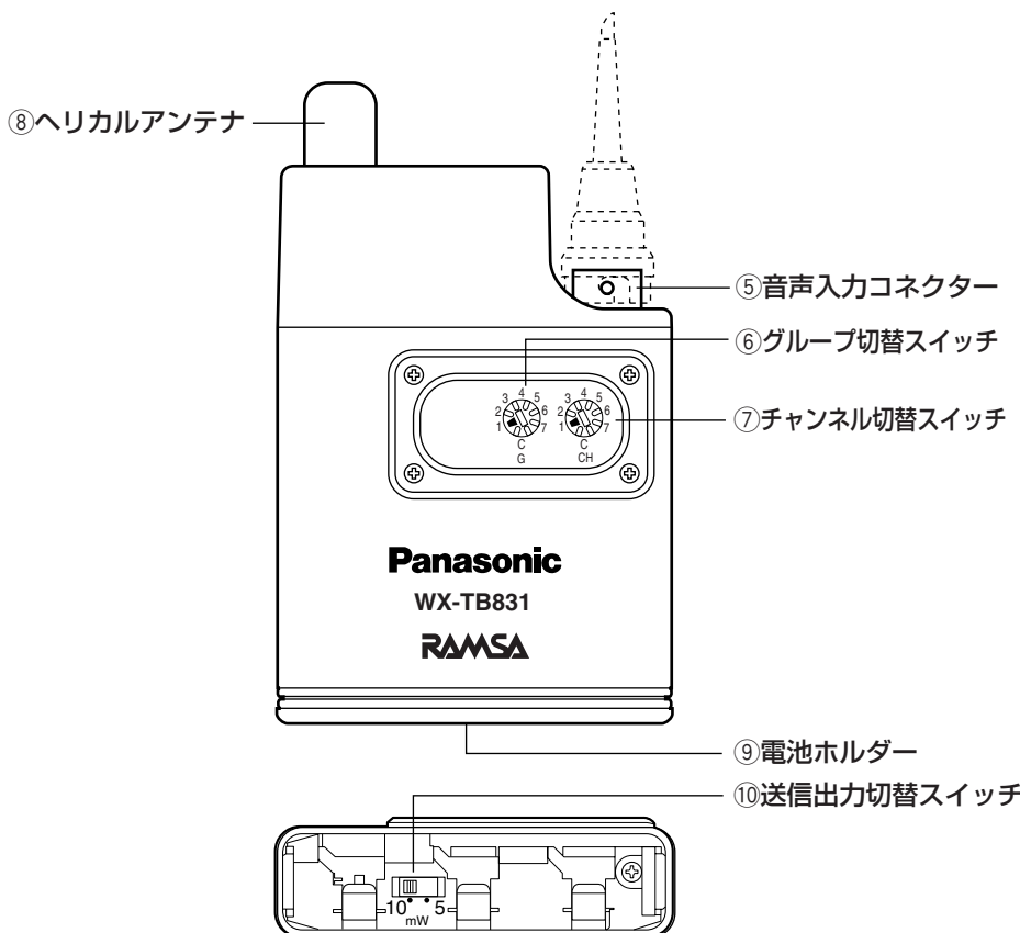
<電池ホルダーを取り外した状態>
