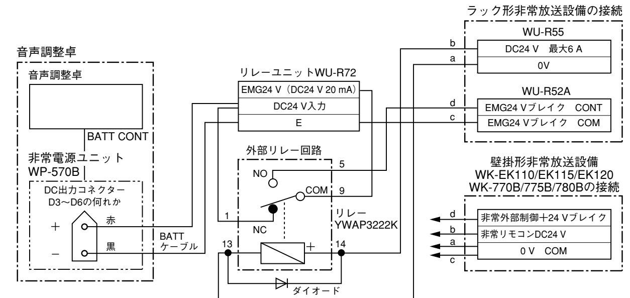
リレー：YWAP3222Kの端子図
