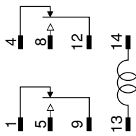
内部結線図
