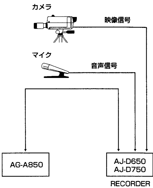
カメラ/外部入力編集
