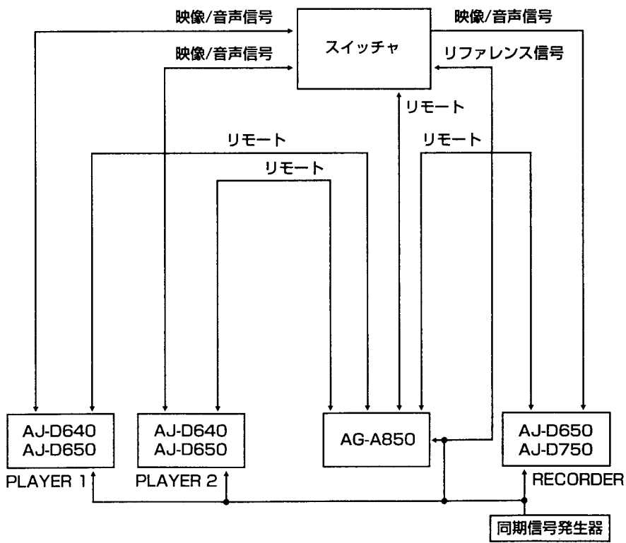
2台の再生機を使つてのシステム (A/Bロール編集)
