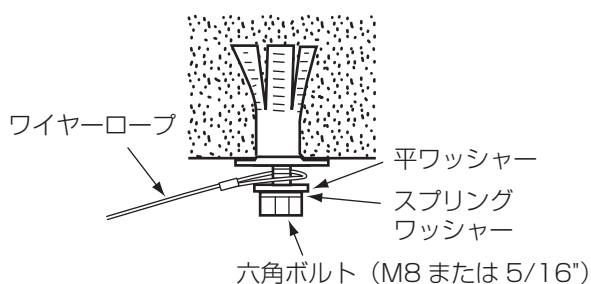
アンカーナット またはカールプラグ (M8 または 5/16")
