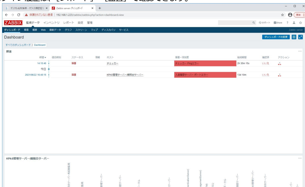
図 76 Zabbix ダッシュボード
