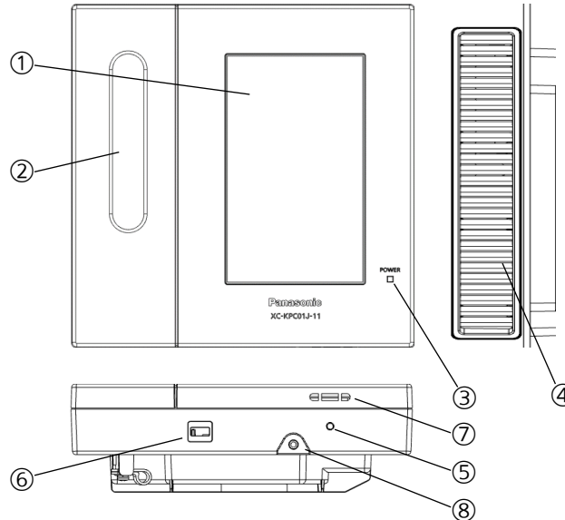
図 2 チェッカー外観
