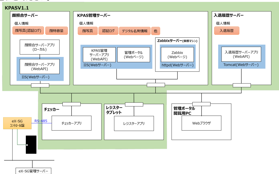
図 1 KPAS システム構成例（ベーシックモデル・入退履歴サーバー単独構成）
