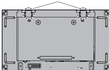
アイボルト取り付け位置
