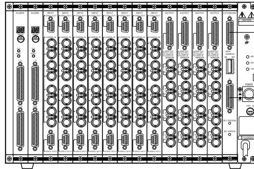
増設ユニット WJ-AD550
