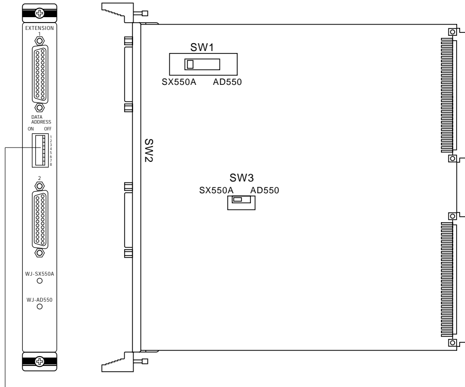
DATAボードアドレススイッチ（操作しないでください）
