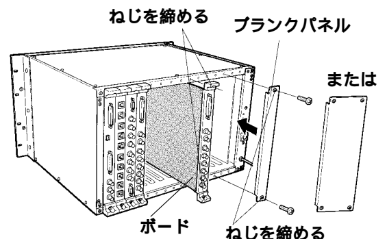
ねじを締める
