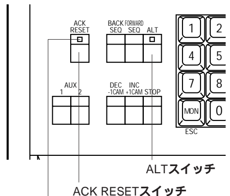
[ACK RESET] スイッチを一回押すと点滅する。再度押すと消える。
