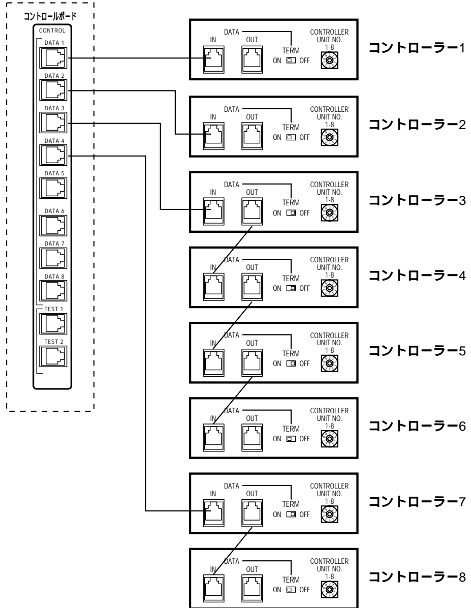
終端とコントローラー番号の設定
