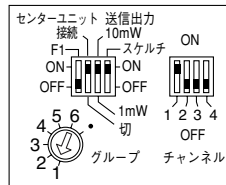
【センタートランスシーバー2】
