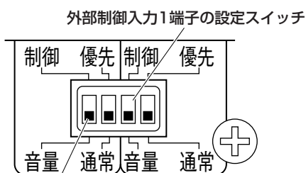
外部制御入力2端子の設定スイッチ
