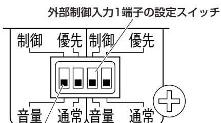
外部制御入力2端子の設定スイッチ
