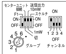
【センタートランスシーバー1】
