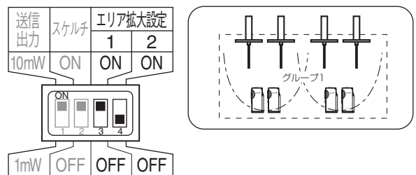
【1グループシステム エリア拡大+同時通話】
