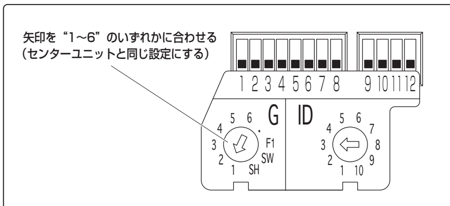
ポータブルトランシーバー裏面
