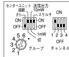
【センタートランスシーバー3】
