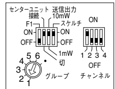
【センタートランスシーバー4】
