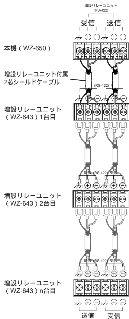
増設リレーユニット接続端子の接続
