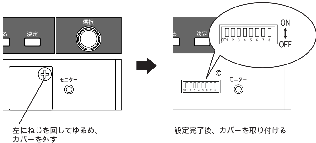
図 設定スイッチ
