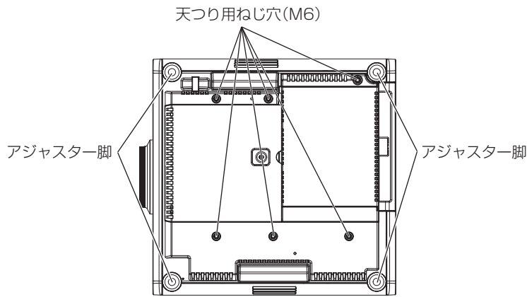
天つり用ねじ穴とアジャスター脚の位置
