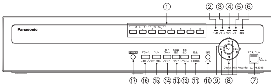
図3：前面パネル
