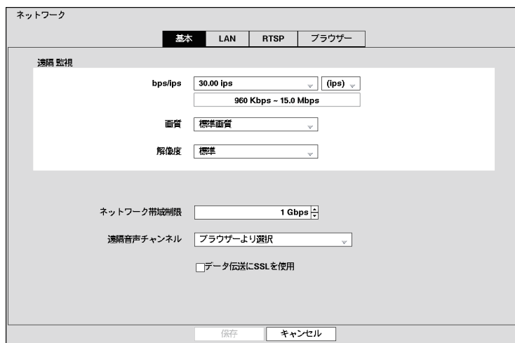
図61：ネットワーク — 基本設定画面
