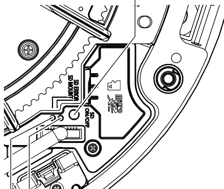
⑤SD ERRORランプ (S857xL) SD ERROR/AFランプ (S854xL)
