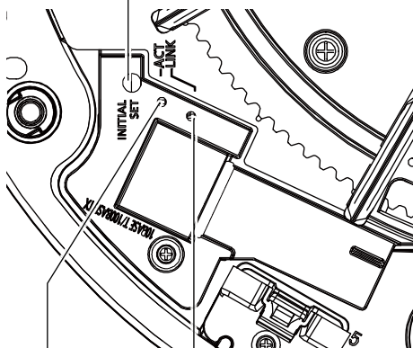
③ACTランプ ②LINKランプ
