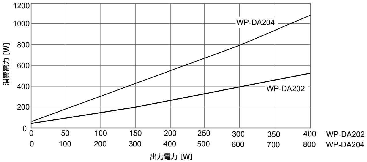
電力特性（全チャンネル出力合計）
