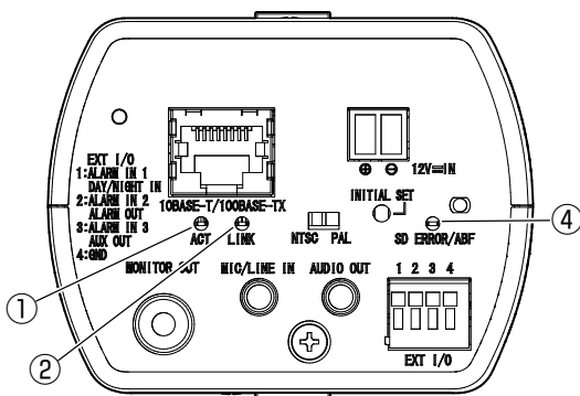
本機背面図
