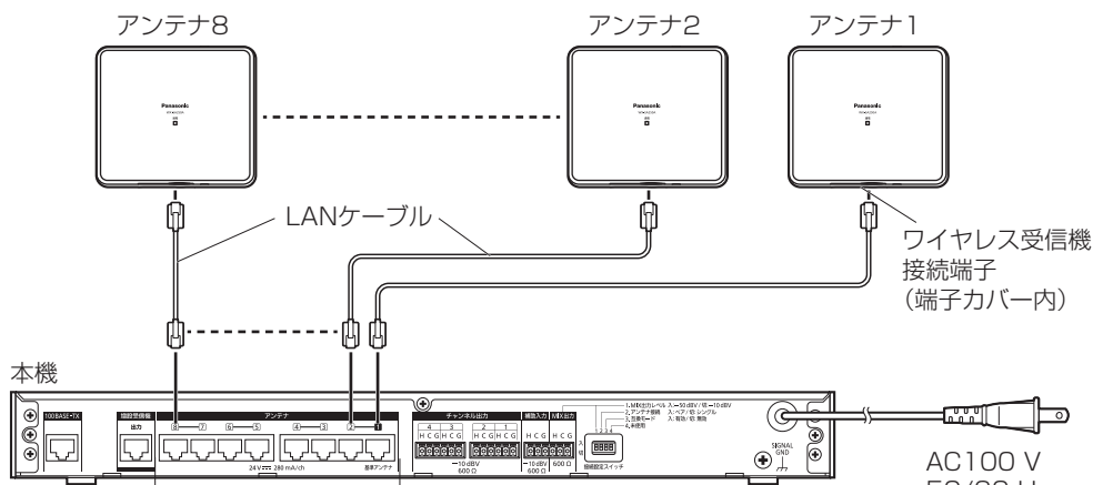
ワイヤレスアンテナ接続端子 1~8
