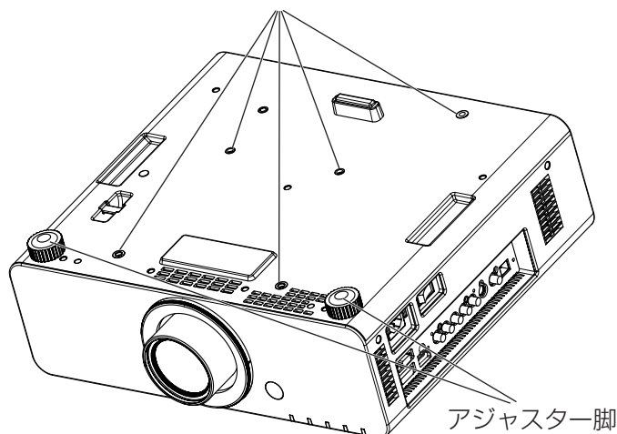
天つり用ねじ穴 (M6)
