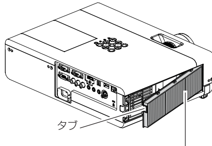
図3 エアフィルターユニット
