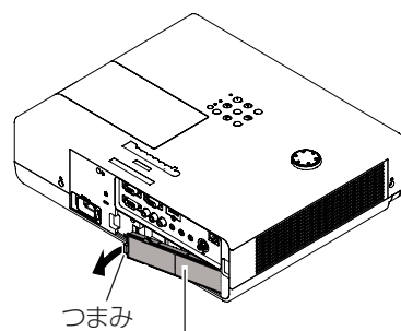
エアフィルターユニット (後面)
