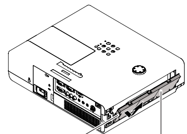
つまみ エアフィルターユニット (側面)
