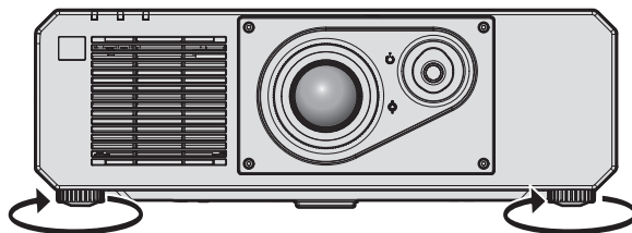
最大調整可能量 各アジャスター脚：35 mm
