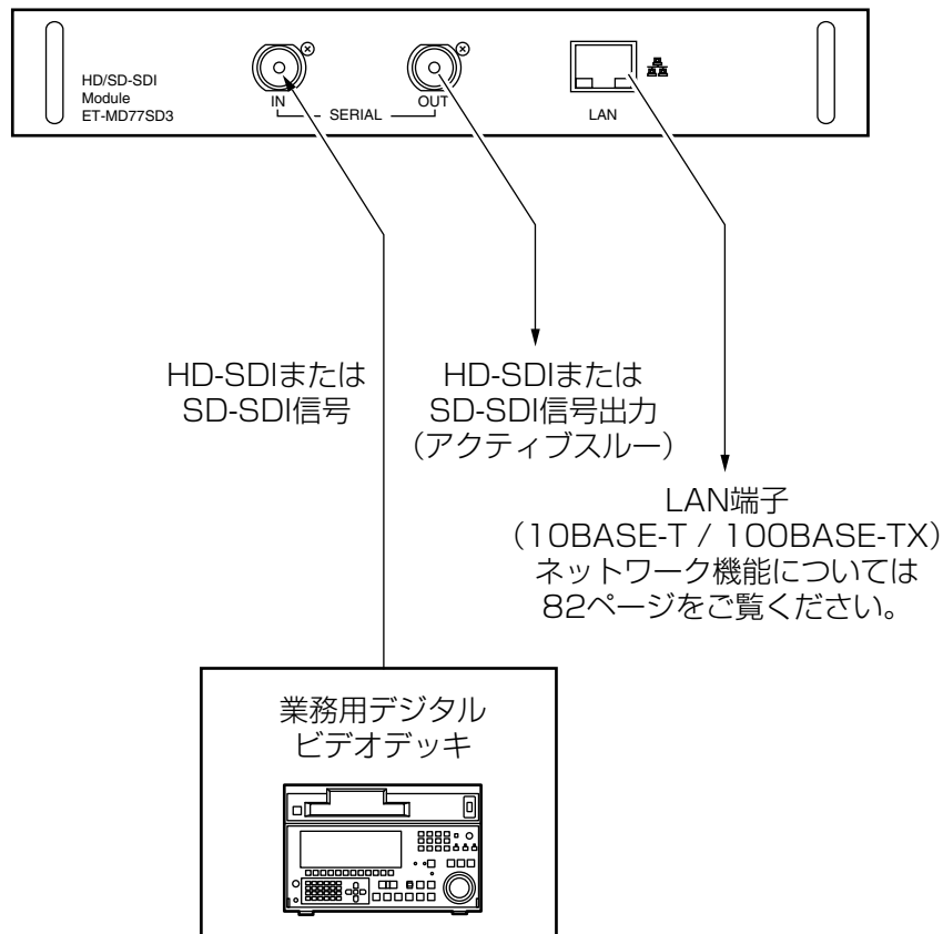
HD/SD-SDI入力モジュール(別売品) ET-MD77SD3 (HD/SD用)
