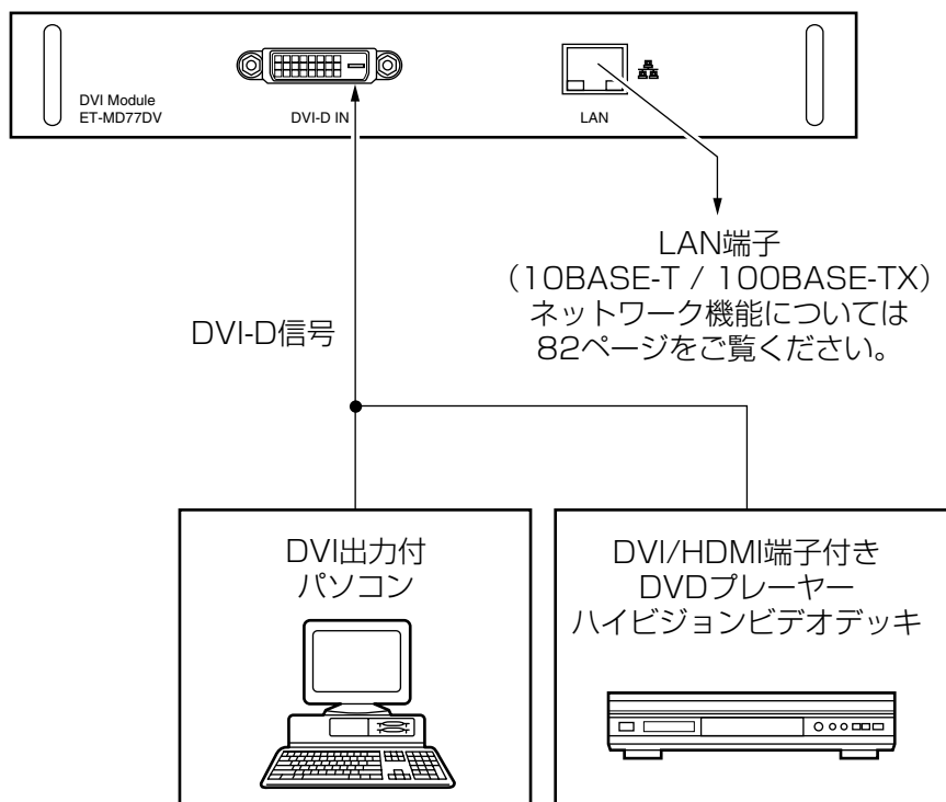
DVI-D入力モジュール(別売品) ET-MD77DV
