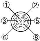
8ピン DIN (外側から見た図)
