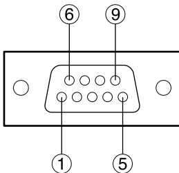
D-Sub 9p (メス) 外側から見た図
