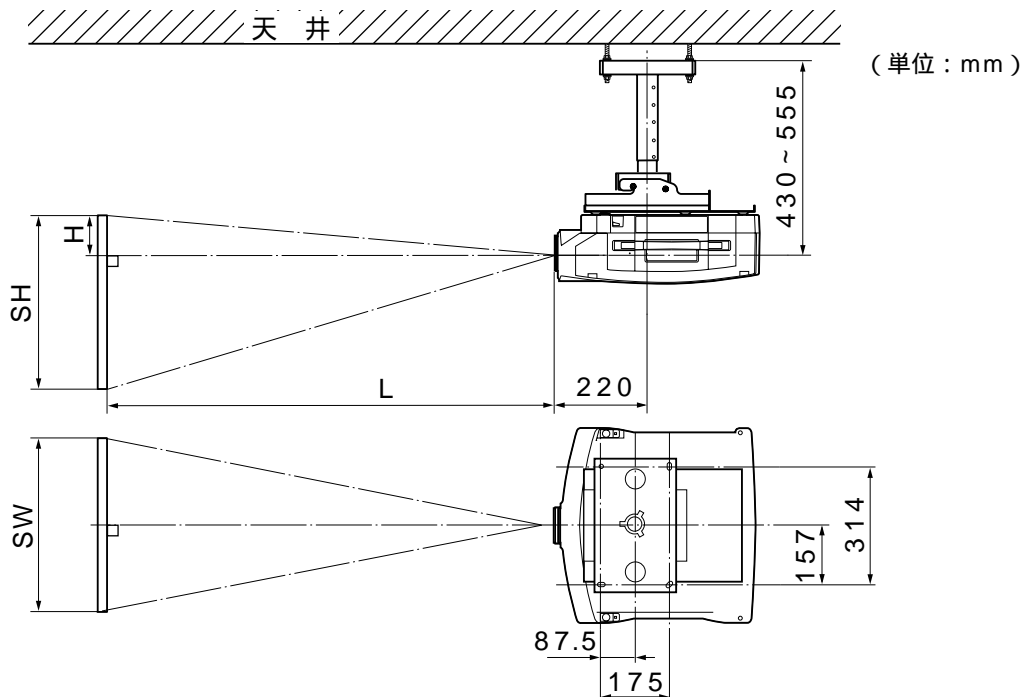
投写関係寸法 (TH-L6500J/TH-L6600Jの場合)
