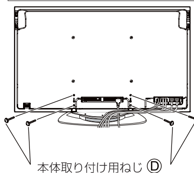
プラズマディスプレイ本体後面
