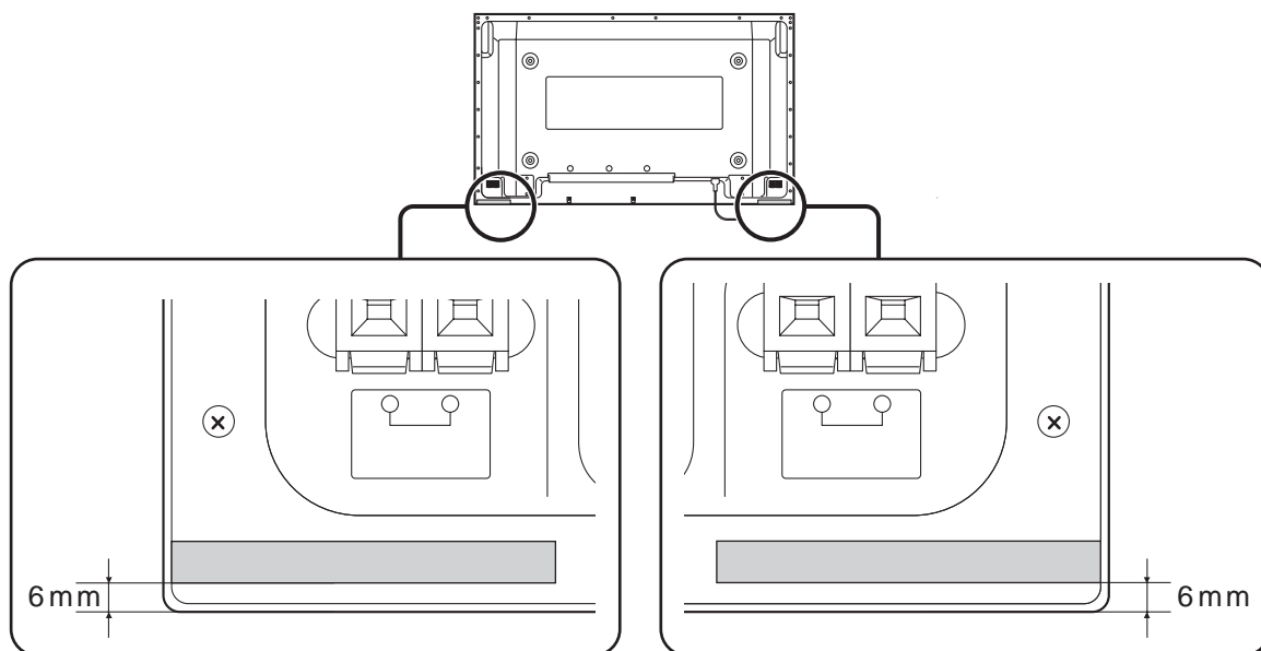
導電テープ貼付位置の目安
