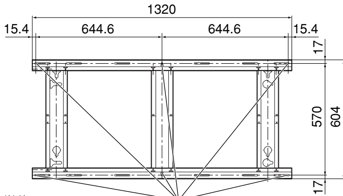
壁面取り付け穴 (6個所)
