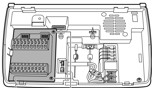
オプションボード（別売り） オプションボード固定ねじ（オプションボードに付属）
