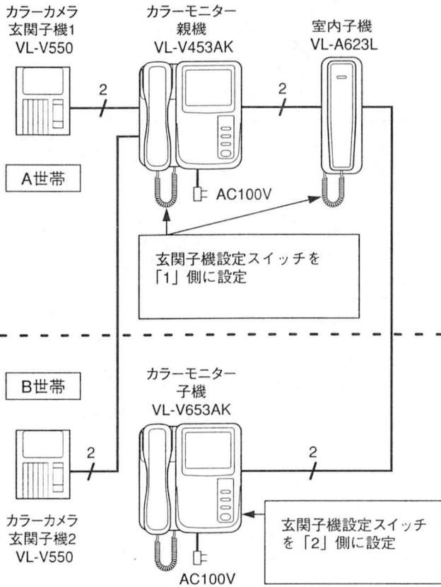
(配線系統図)
