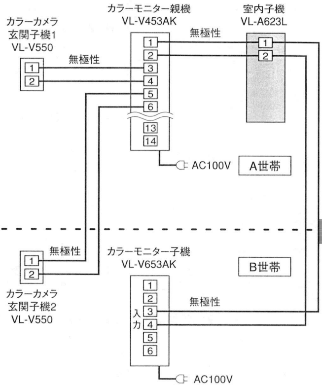
(接続図)
