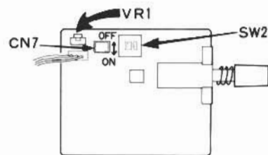
コールサイン基板(部品取付面)
