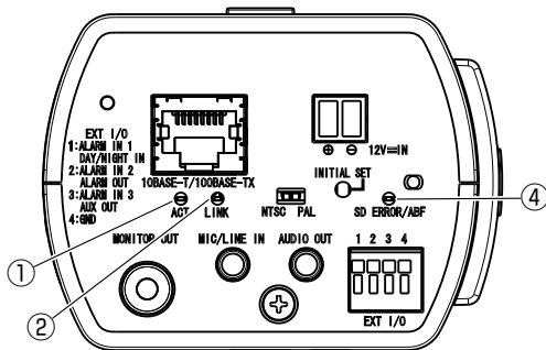
本機背面図
