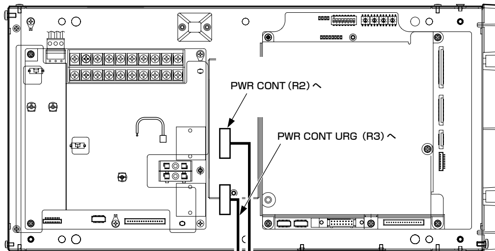
非常リモコン WR-EC500 パネルを開いた図
