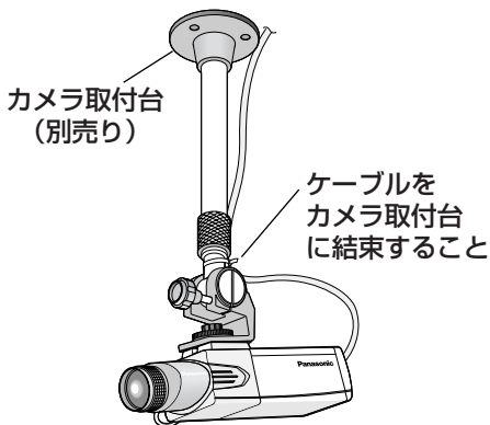
<天井へのカメラ設置例>
