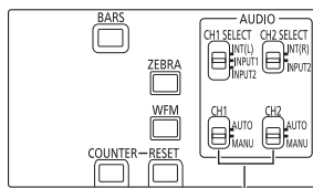
AUDIO AUTO/MANU CH1, CH2 スイッチ
