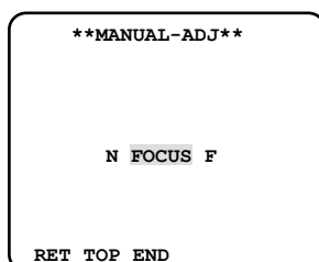
「MANUAL-ADJ」画面
