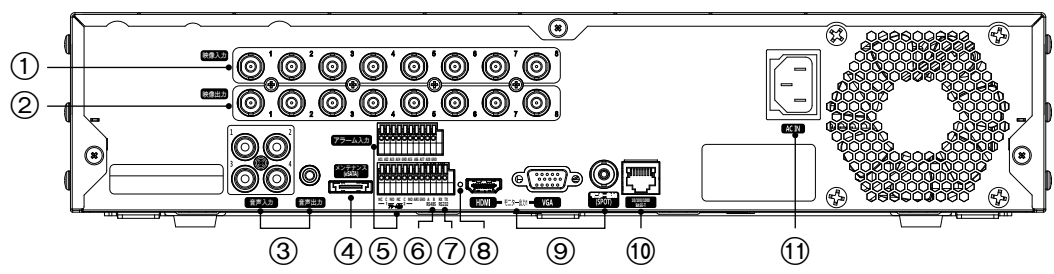
図2：本体後面図
