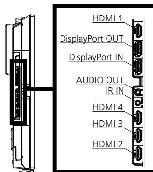
端子部拡大図 a
